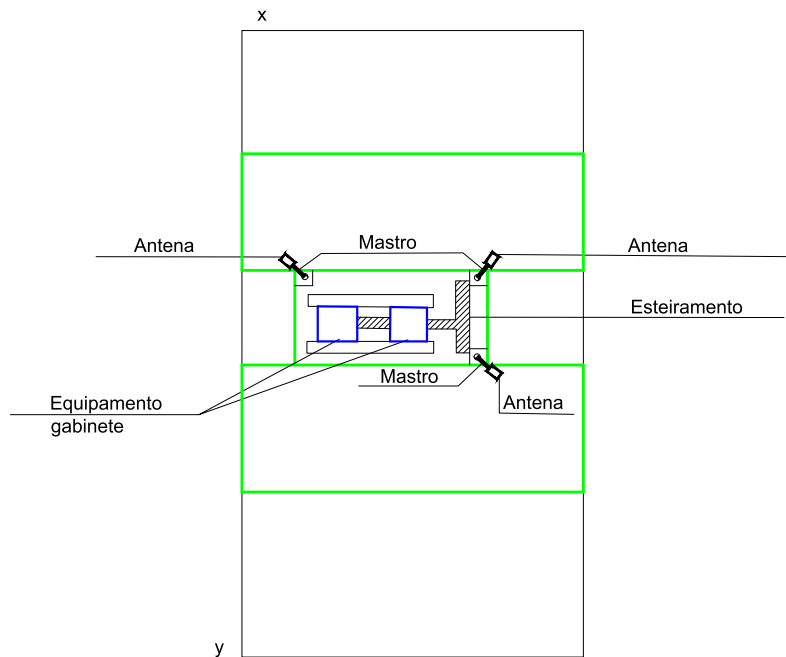
Implantação esquemática esc.
